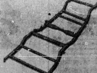
Robustes châssis de type échelle à longerons latéraux en U et traverses en mécano d'alligatox.
