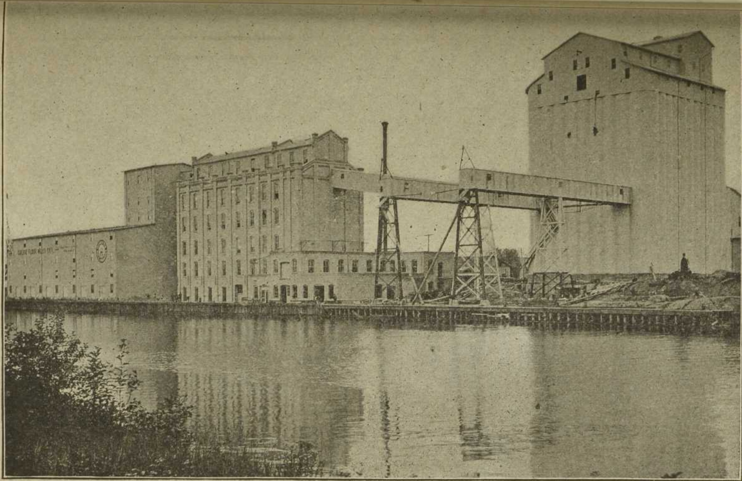
MOULINS DE FORT WILLIAM. CAPACITÉ 4000 BARILS PAR JOUR. THE OGILVIE FLOUR MILLS COMPANY LIMITED, FORT WILLIAM, ONT.
