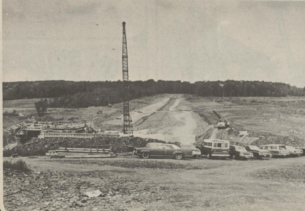
Une vue d'ensemble du projet. La construction présente le puits de contrôle et les déversoirs. A l'arrière-plan, le chantier de construction de la digue principale.
