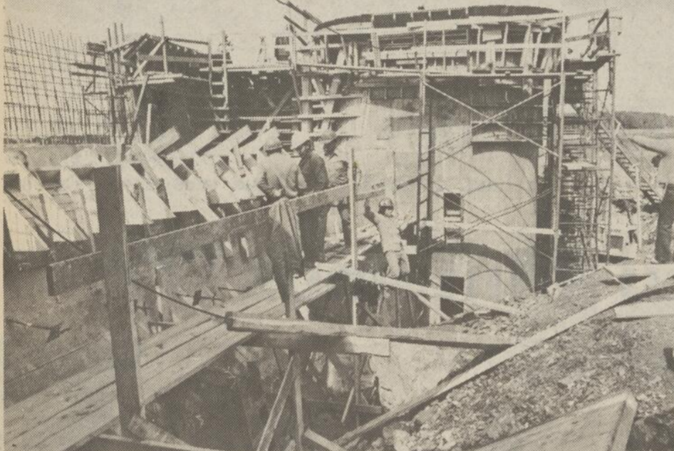
A l'extrémité de la digue principale, on retrouve les déversoirs gauche et droit et le puits de contrôle.
