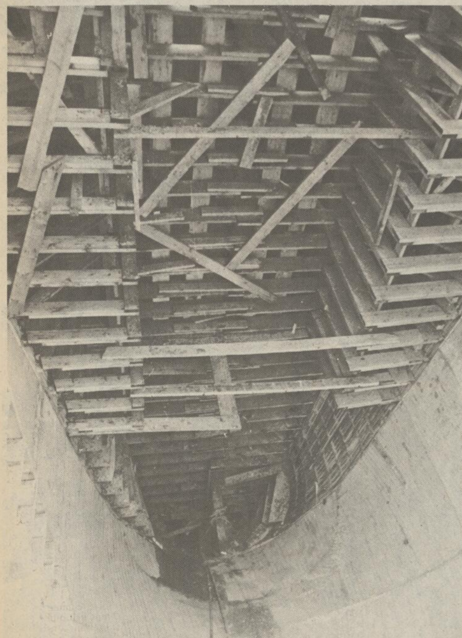
Le puits de contrôle n'est pas encore tout à fait terminé. Sa profondeur: 72 pieds.
