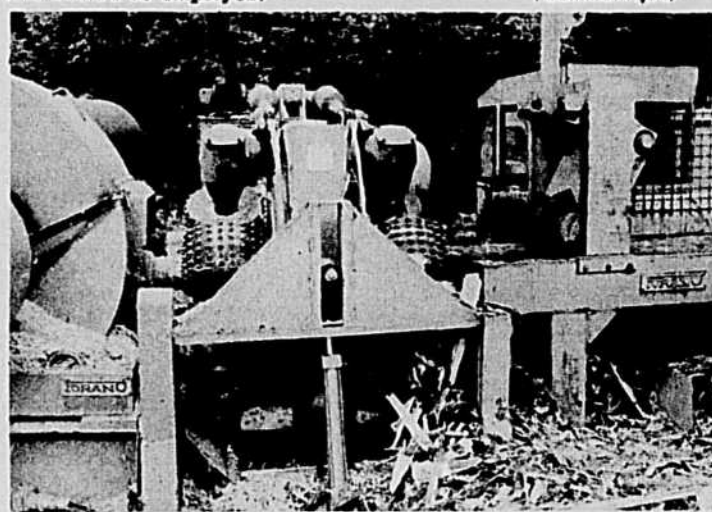
Déchetage en forêt - Vue de côté de la nouvelle déchiqueteuse mobile de Domtar Limited, qui transforme les billes en copeaux en pleine forêt. A droite, le convoyeur pousse une bille à travers l'écorceuse au centre jusqu'à la déchiqueteuse à gauche. Cette nouvelle machine, fruit de la recherche des spécialistes de Domtar, subit présentement des essais dans les Cantons de l'Est.
