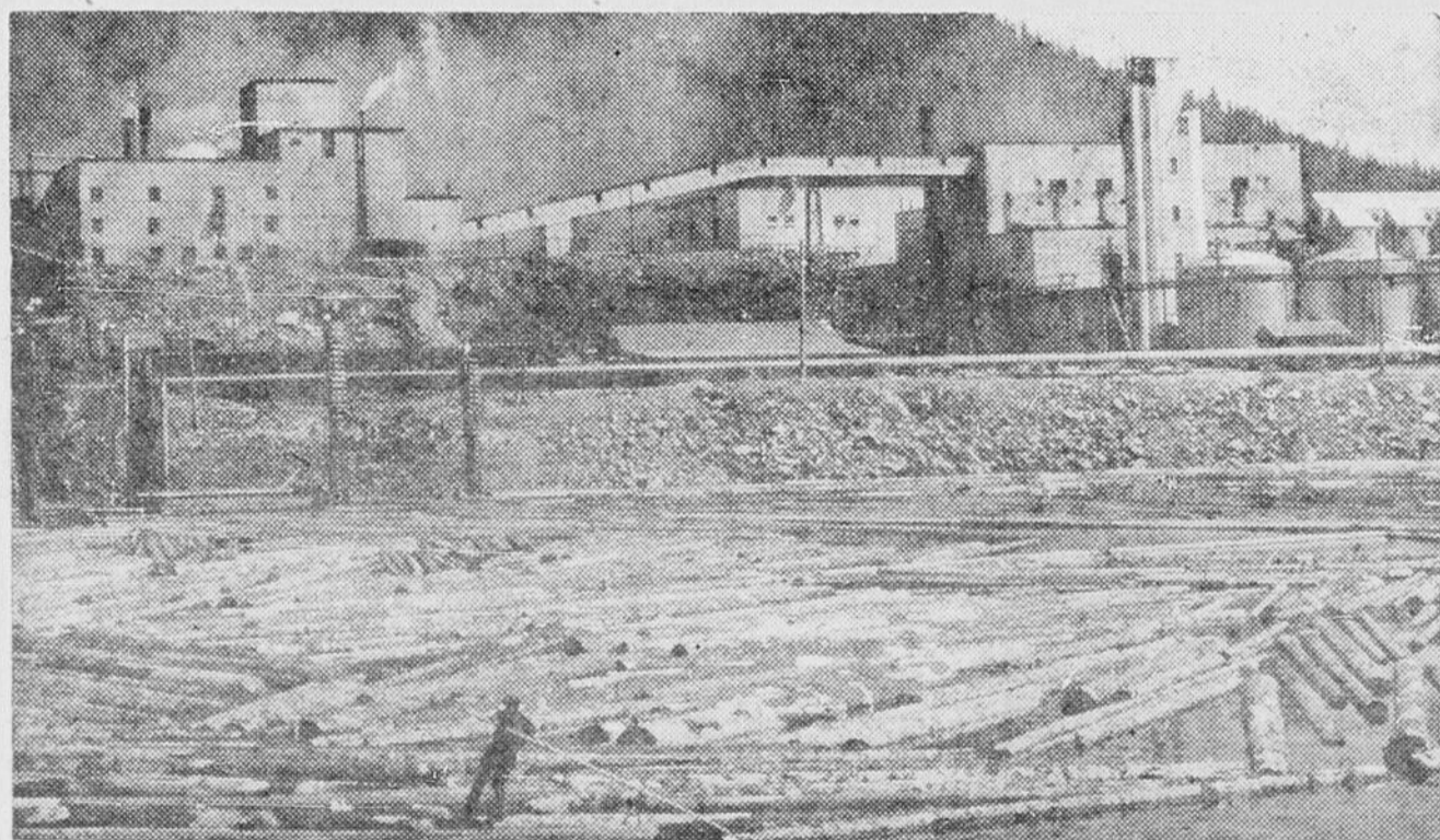
Cette usine, située sur l'île Watson, Colombie-Britannique, sert uniquement à la fabrication de la cellulose. Les billes de bois sont coupées en petits morceaux, placés ensuite dans une des six "marmites" d'une capacité de 50 tonnes, orgueil de l'usine, où ils bouillent jusqu'à leur transformation. L'usine est reliée aux grands centres du Canada et des États-Unis par rail, et par son port de mer, libre de glaces à l'année longue. (Photos de l'Office national du film du Canada, par Gar Lunney.)
