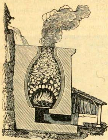
FOUR À CHAUX
