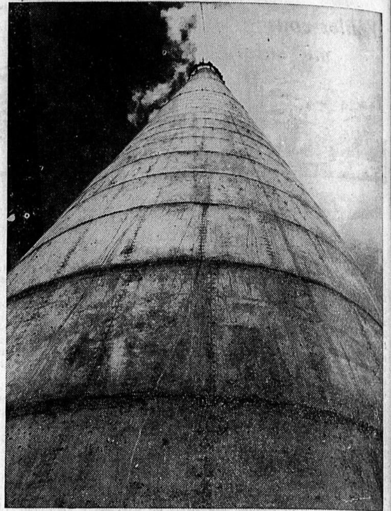
• Aperçu d'une cheminée de 400 pieds de hauteur lorsqu'on est placé à sa base. Cette cheminée, la plus haute de toutes les cheminées desservant les cimenteries de l'Amérique du Nord, vient d'être construite pour les Ciments du St-Laurent. (St-Lawrence Cement Company) à Ville-neuve, près de Québec.
