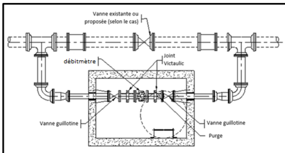
Figure 6. Installation d'un débitmètre sur une conduite en dérivation
