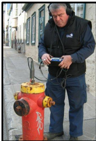
Figure 8. Écoute sur un poteau d'incendie
