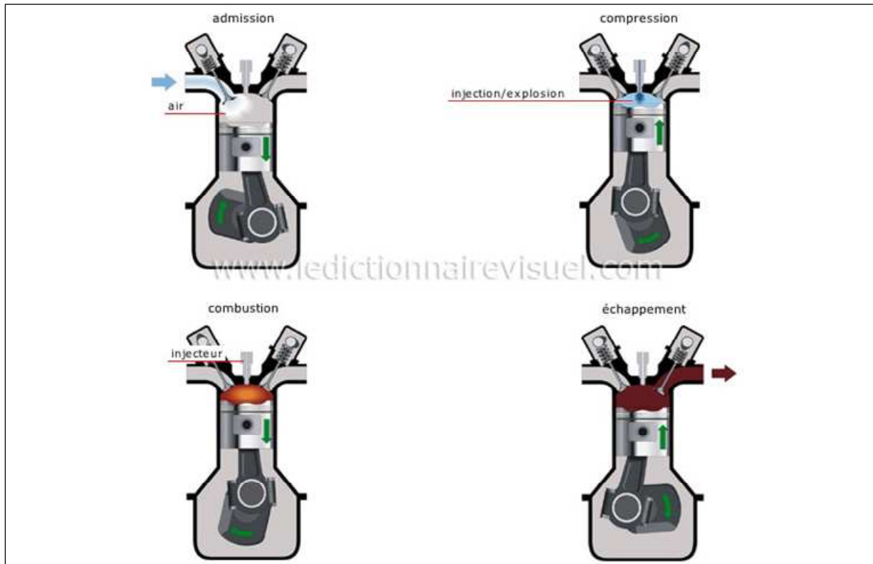
Figure 7 Illustration du cycle d'un moteur diesel
