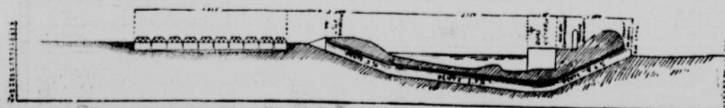
Section longitudinale du tunnel projeté pour relier Montreal à la rive Sud
