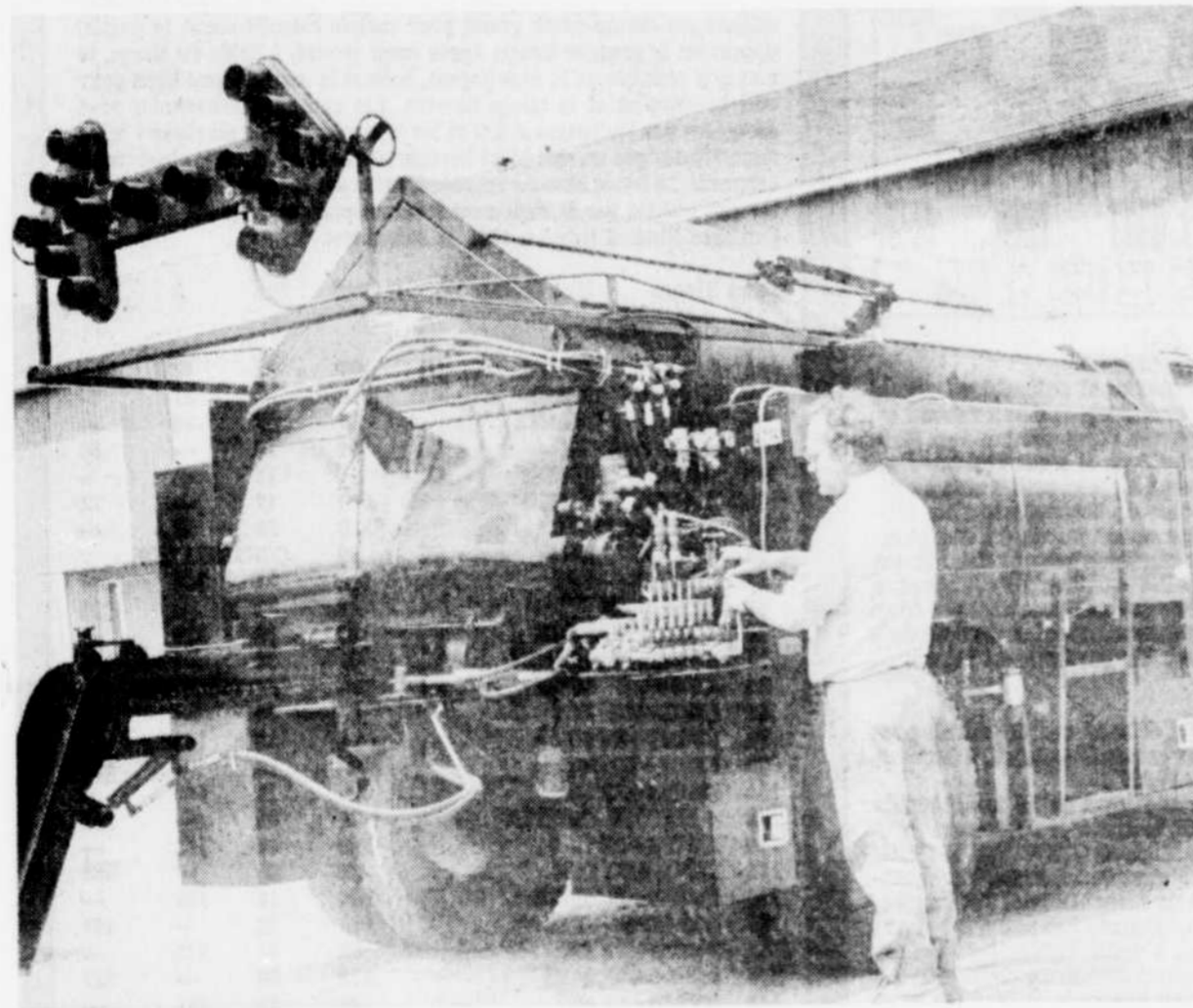
La ville de Thetford Mines s'est portée acquéreur du premier prototype de ce nouvel épandeur d'asphalte, entièrement hydraulique.
