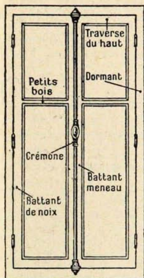
FIG. 77.—Fenêtre.
