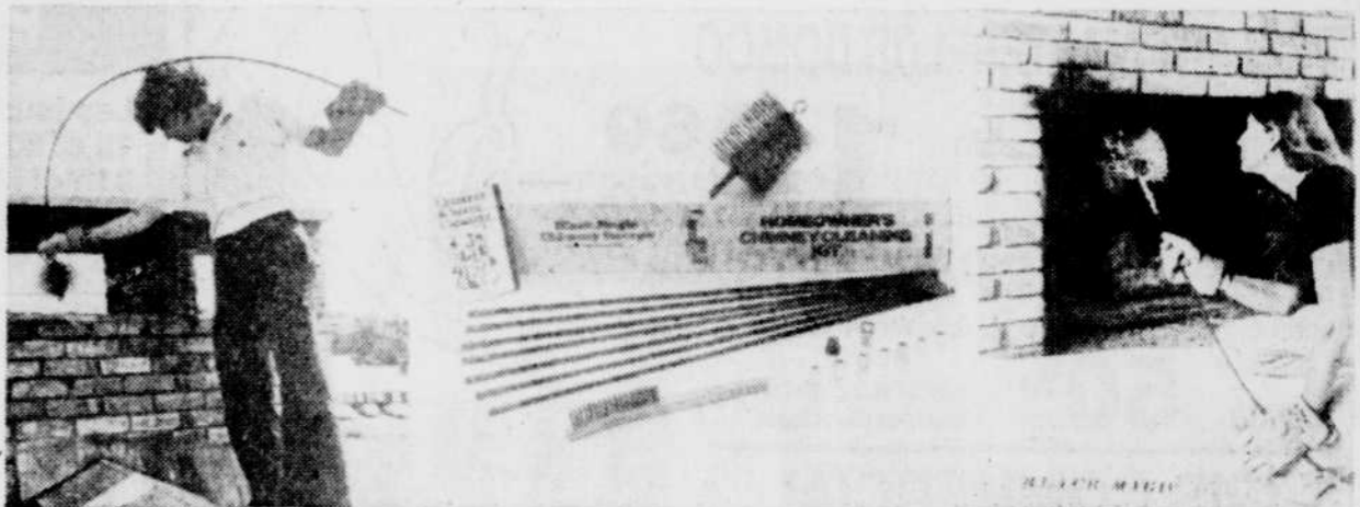
Un nécessaire complet qui permet au propriétaire d'une maison de faire lui-même le ramonage de la cheminée.
