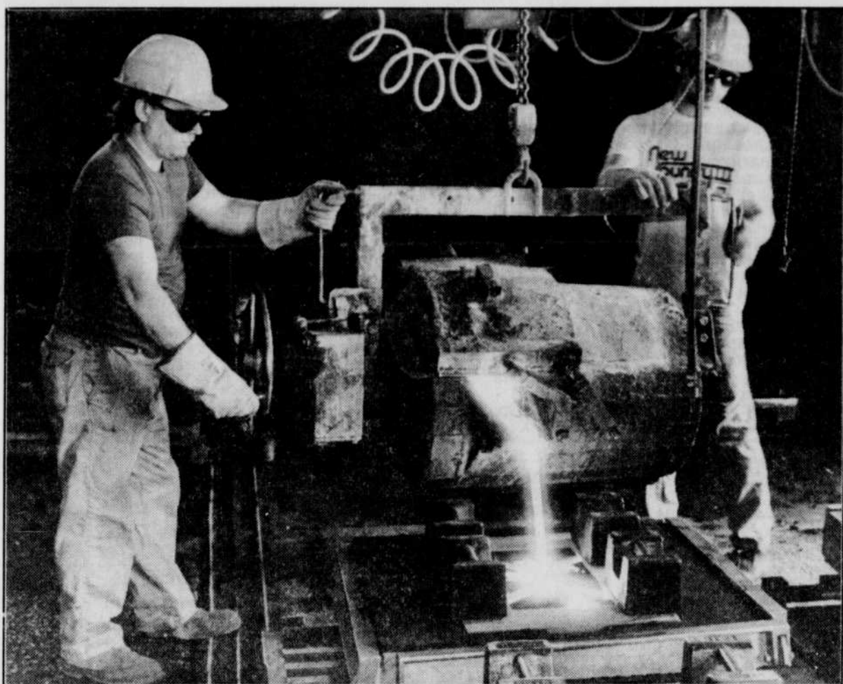
La fonte au cubilot est une chose du passé. Maintenant, c'est le système par induction qui a pris la place. En 30 minutes, les fondeurs peuvent effectuer une coulée.
