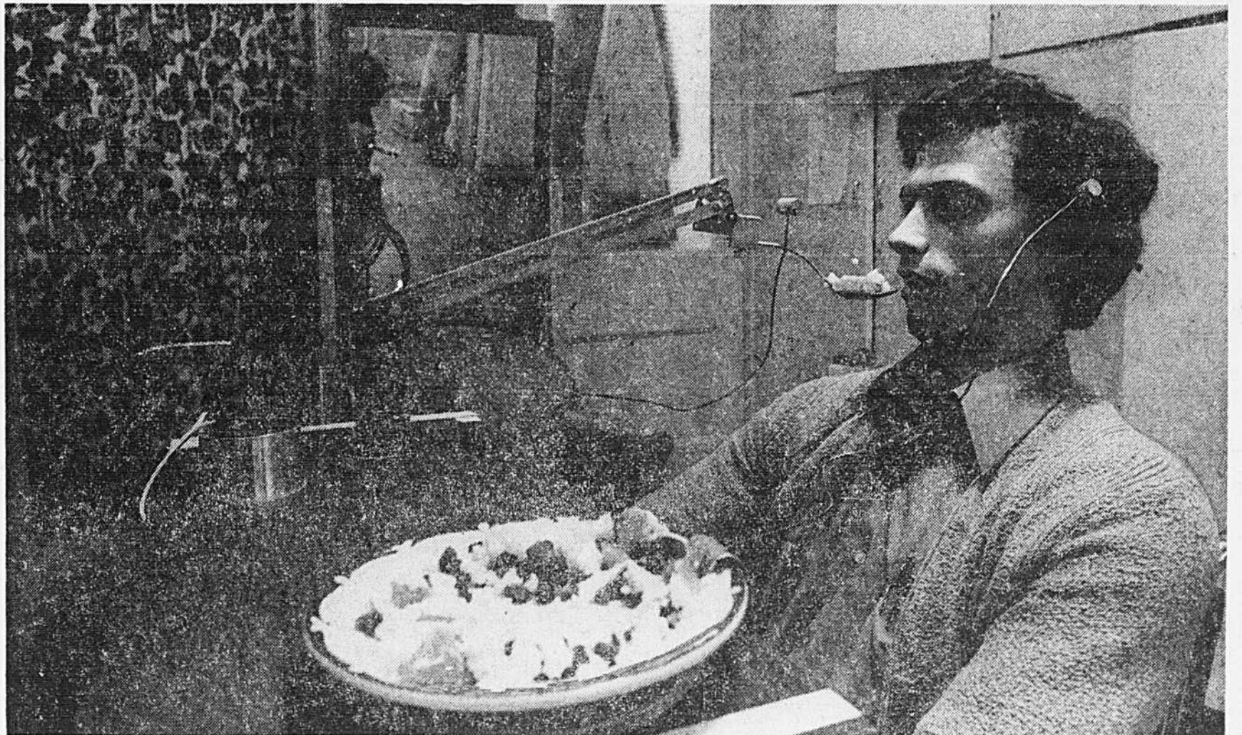
Douglas Kennedy, un des trois inventeurs de "l'alimenteuse automatique", démontre ici comment cette machine permet à une personne paralysée de la nuque aux pieds de se nourrir sans assistance. La cuillère plonge dans l'assiette, sur commande, se remplit d'aliments, déverse son trop plein et remonte automatiquement vers la bouche du malade.
