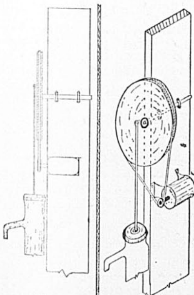
VUE DE FACE - VUE ISOMÉTRIQUE
