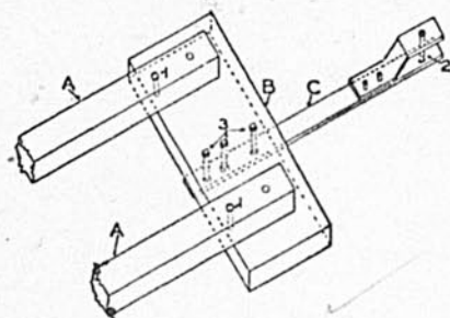
VUE ISOMÉTRIQUE.
