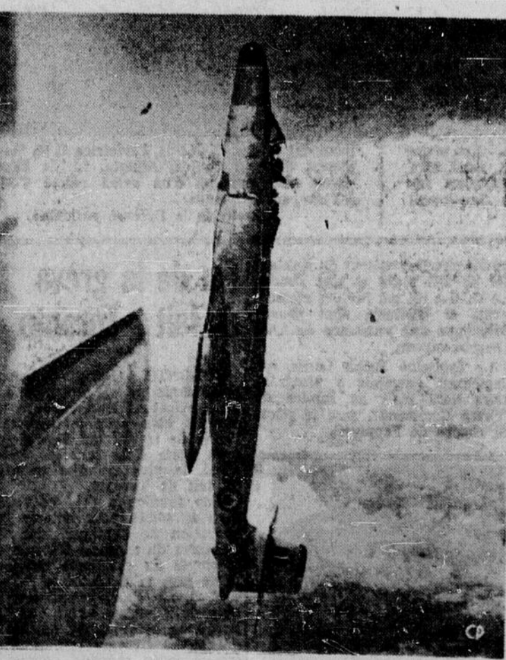
LE CF-100 POUR LE LANCEMENT DE FUSEES — Voici la première photographie du dernier modèle du CF-100 que l'on considère comme l'avion de combat le plus fortement armé au monde. On voit ici l'appareil en montée verticale. On peut très bien distinguer les porte-fusées à la pointe des ailes. Aujourd'hui, on produit cet appareil en série aux usines de l'A. V. Roe (Canada) Limited, à Malton, banlieue de Toronto, pour le C.A.R.C. (Photo P.C.)
