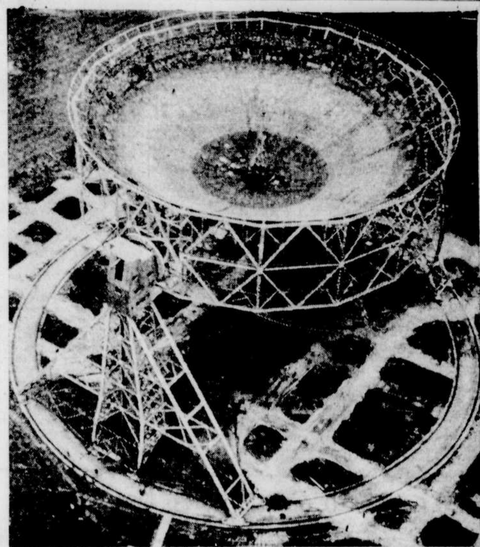
Le radio-télescope de Jodrell Bank, en Grande-Bretagne
