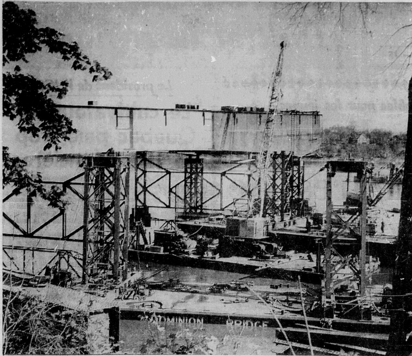
EXPLOIT DE CONSTRUCTION — Comment transporter une travée de 1,500 tonnes de Hull à Ottawa sur la rivière Outaouais, c'est l'exploit que devront réussir, vendredi matin, les ingénieurs de la compagnie Dominion Bridge. Pour cela,
