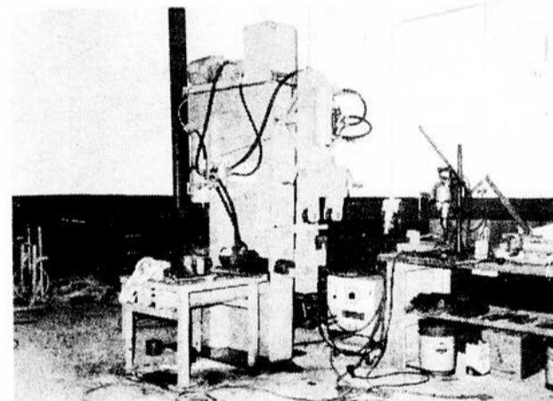
Notre nouvelle acquisition; notre table d'assemblage et plieuse d'oeil de ressort et pour arquer les lames.
