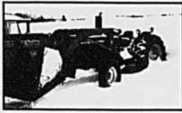
John Deere 1020, gaz, moteur refait à neuf. Très bonne condition 4,800 $
