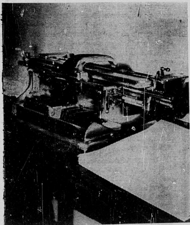
Machine à transcrire en braille
