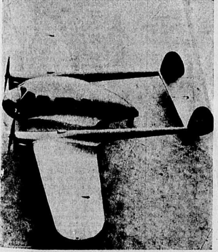
Voici la réplique américaine au "Pou-du-ciel" d'invention française. Il s'agit, comme le démontre cette photo, d'un petit monoplane d'une ligne très audacieuse et entièrement nouvelle. Tout le fuselage est consacré à l'espace réservé aux passagers. Les moteurs sont placés dans deux membres parallèles qui vont en s'écartant vers l'arrière. Ces moteurs donneront une vitesse maxima de 230 milles à l'heure à cette minuscule nacelle construite par la "American Gyro Company" de Denver. L'avion ne consomme que 11 gallons de gazoline à l'heure et à peu près une chopine d'huile à moteur. On l'appelle le "Crusader". Cette photo fut prise à l'aéroport de Burbank, Californie.
