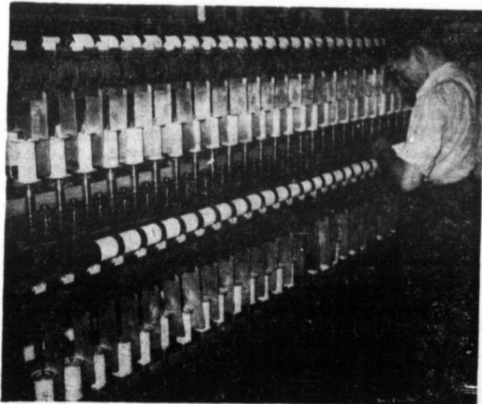
LE "TWISTAGE" — C'est l'opération qui consiste à enrouler ensemble plusieurs fils de nylon pour en former un plus résistant...
