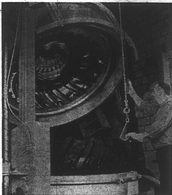
Sur le point d'être retiré de son moule à l'usine de Toronto, ce pneu Goodyear est le plus récent qui soit destiné à l'industrie forestière. Désigné comme le pneu Timber Torque Steelguard, il est renforcé de deux couches de fil d'acier sous la bande de roulement, ce qui pratiquement élimine les crevaisons. Ce pneu mesure plus de six pieds de diamètre et pèse environ une demi-tonne.
