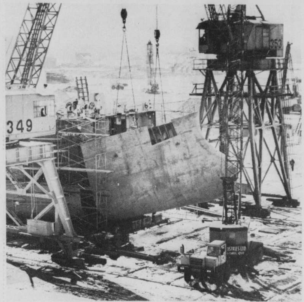
Il en a coûté $250,000 à l'Imperial Oil pour refaire la toilette de son pétrolier des Grands Lacs Imperial London, construit il y a vingt ans. Parmi les travaux en cours aux Chantiers de Sorel de Marine Industrielle, selon les derniers principes de l'architecture maritime, mentionnons l'installation d'un bulbe à la proue et la réfection de l'arrière selon des lignes aéro-dynamiques, en vue d'accroître la rapidité et le rendement du bâtiment. Dans la photo, des ouvriers mettent en place la proue renflée. (Photo de l'Imperial Oil)
