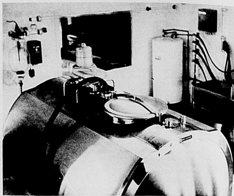
L'utilisation d'un bassin réfrigérant moderne est un atout précieux pour le producteur mais son utilisation exige des vérifications régulières et systématiques pour que la qualité du lait soit préservée.
