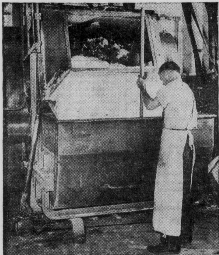
La pulpe arrive à l'usine en grandes feuilles, trempe quelque temps dans un acide, est asséchée, puis passée par cette machine qui la réduit en miettes.
