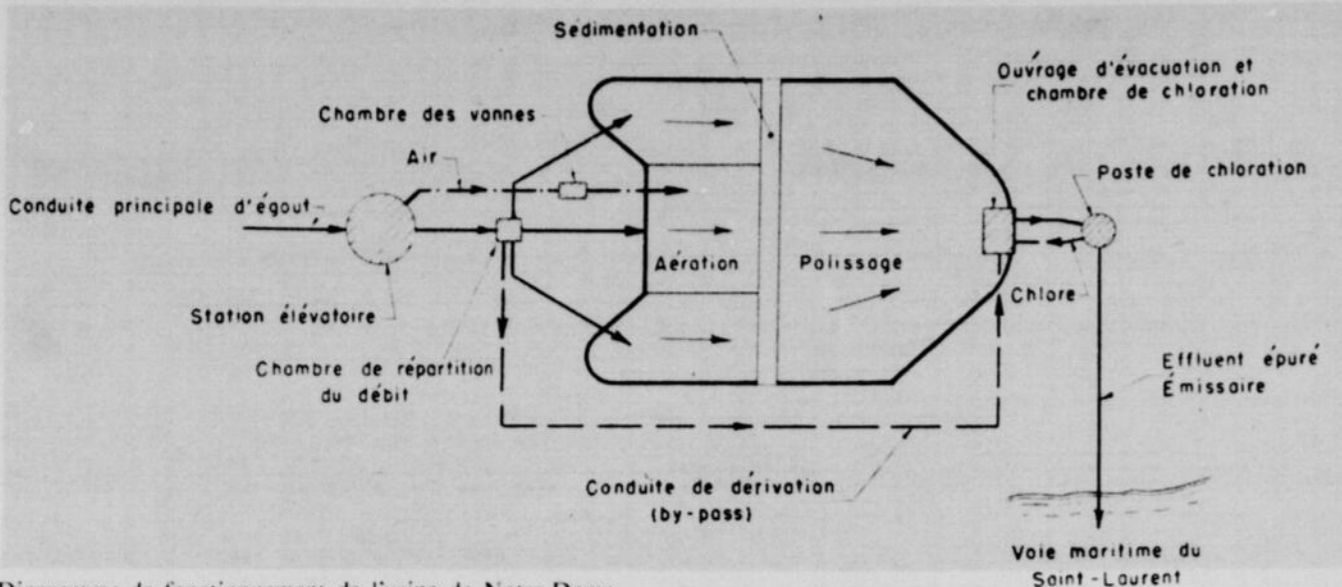
Diagramme de fonctionnement de l'usine de Notre Dame.
