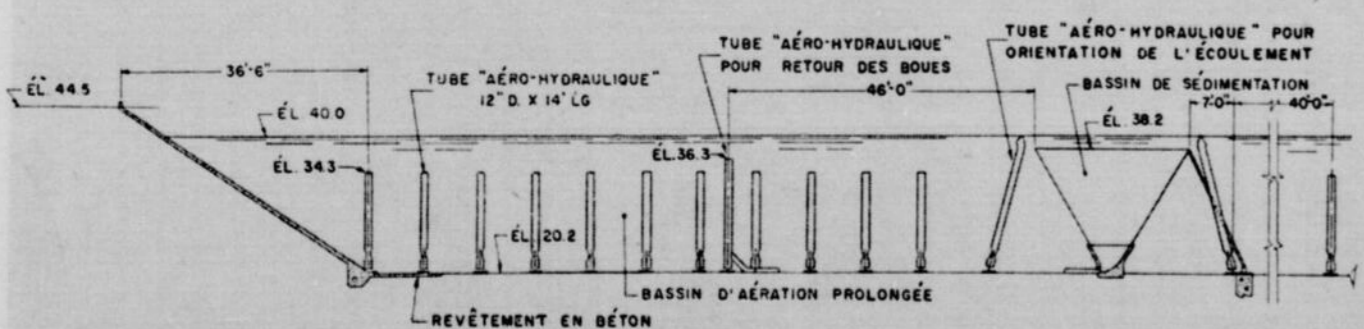
Coupe du bassin de l'usine d'épuration de Notre Dame.
