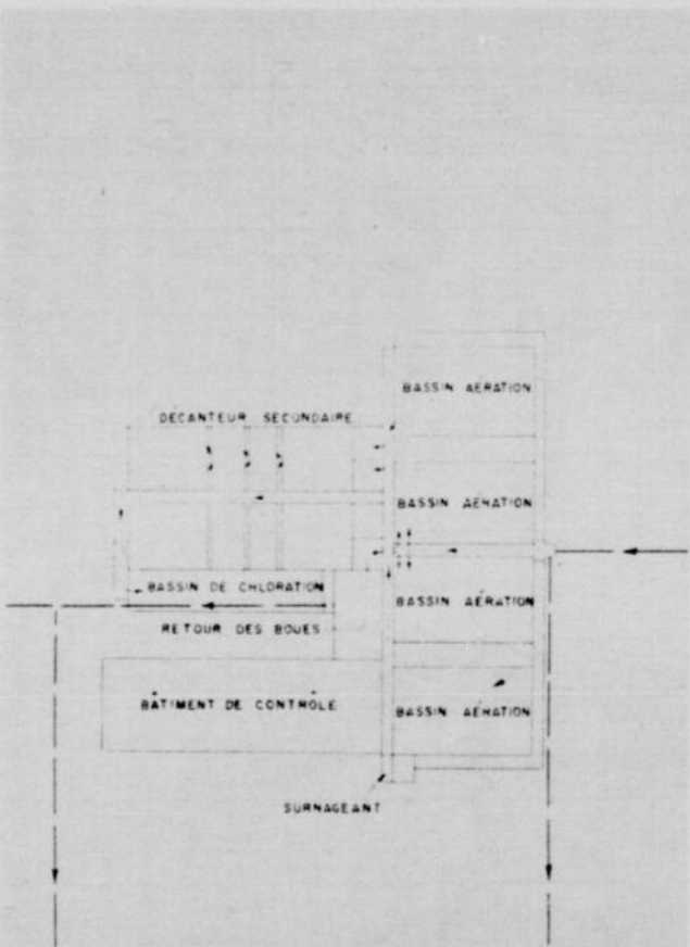
Diagramme de l'usine d'épuration de McKaye.
