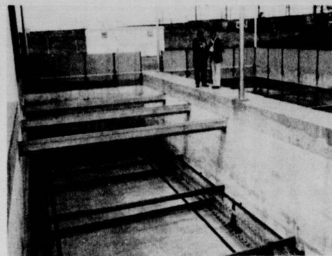
L'un des deux bassins de décantation secondaire, à vide, à l'usine de McKaye. Au fond du bassin, des pales fixées à des chaînes motrices pour la récupération des boues.
