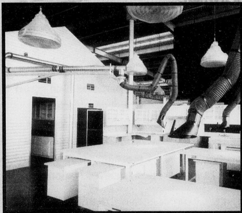
Au-dessus des tables de travail, de grands tuyaux, appelés familièrement « trompes d'éléphant », sont munis d'une lampe et d'un évent puissant qui aspire les vapeurs nocives. Photo des Archives nationales du Canada.
