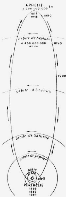
L'orbite de la comète de Halley (dessin gracieusement fourni par l'AGAA).
