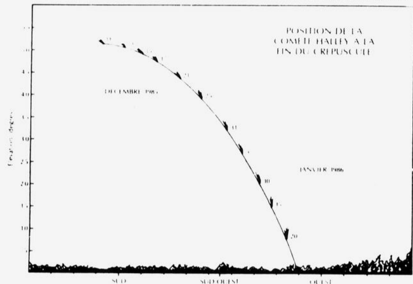
Position de la comète de Halley à la fin du crépuscule, environ 90 minutes après le coucher du soleil (Tiré de la brochure «La comète Halley», publiée par l'AGAA, Montréal, 1985).
