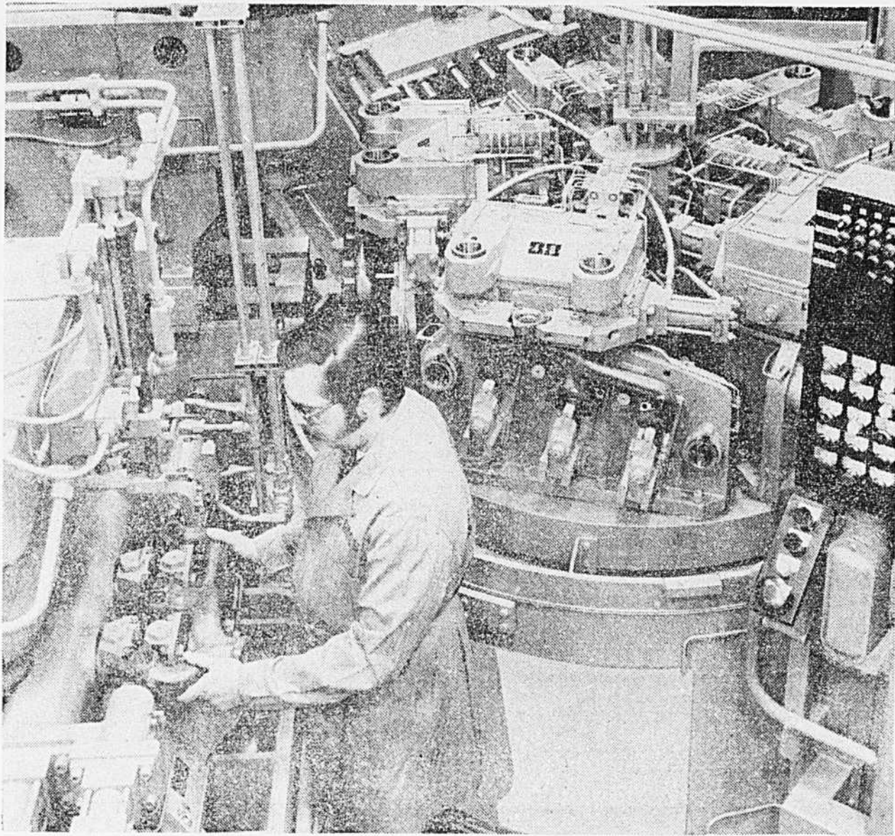
Une nouvelle machine fait tout le forage et tout le polissage d'un collecteur de gaz d'échappement d'automobile, produisant 136 pièces à l'heure.
