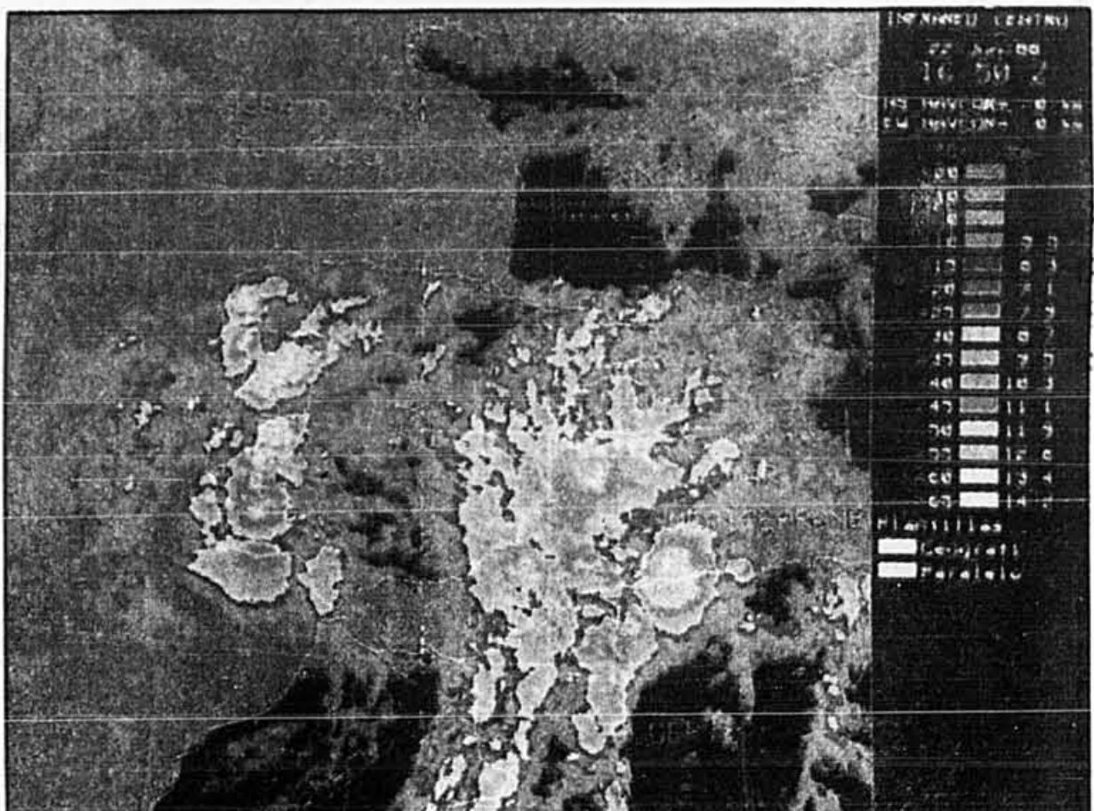
Un satellite a analysé par lumière infrarouge le ciel d'Espagne. La couleur jaune représente des températures de -30 à -40 degrés Celsius, ce qui correspond à des nuages situés entre 8 et 10 kilomètres du sol.
