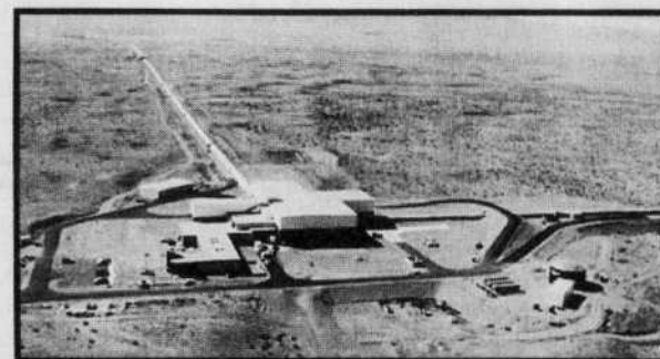
Une vue aérienne du détecteur LIGO situé à Hanford, dans l'état de Washington. Les deux bras du LIGO mesurent chacun quatre kilomètres
