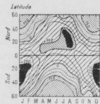
Le bilan radiatif du système Terre-atmosphère: ce schéma représente la différence entre l'énergie solaire reçue par l'atmosphère et la terre et l'énergie qu'elles rayonnent dans l'infrarouge. Elle montre qu'il existe en permanence un excès d'énergie aux latitudes tropicales.
