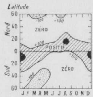
Energie disponible pour alimenter la circulation générale des masses d'air et des courants marins: il existe toute l'année un large excès d'énergie libre dans les régions équatoriales, ce qui explique que des masses d'air équatoriales se déplacent constamment en direction des régions polaires et que les courants marins accomplissent un trajet analogue.
