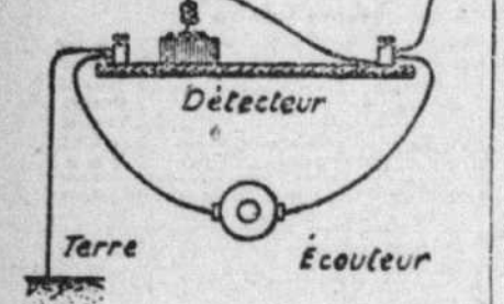
Fig. 8.—Montage d'un poste de T.S.F. avec détecteur à galène
