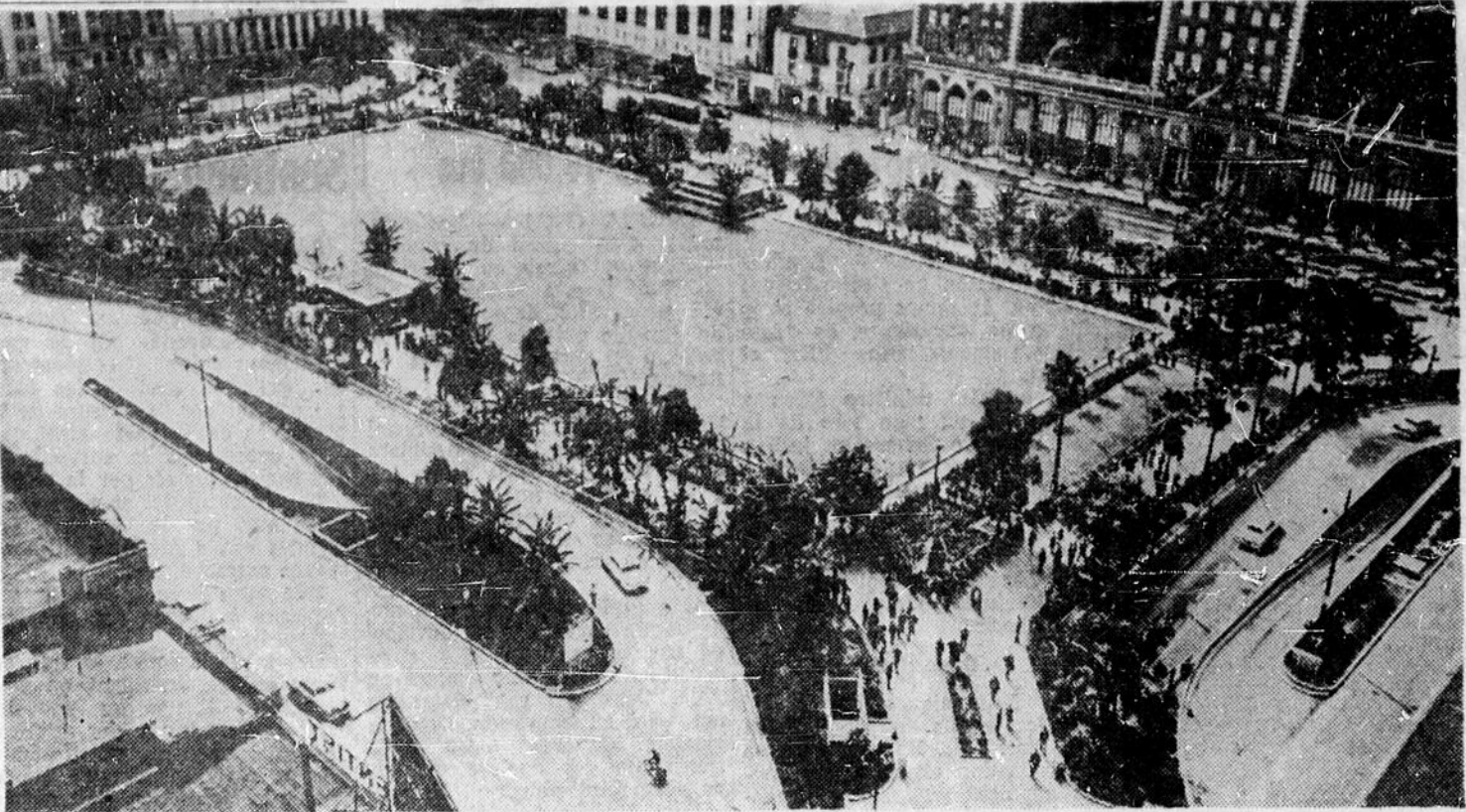
UN VASTE GARAGE SOUTERRAIN — Sous le carré Pershing à Los Angeles, un organisme privé a aménagé un garage de stationnement de trois étages d'une capacité de 2,800 véhicules. Celui-ci en plus d'aider à la solution du problème du logement, rapporte $80,000 de loyer à la municipalité et pourra servir d'abri en cas de guerre. L'échevin Wilbert Hamilton en préconise de semblables à Ottawa. (Cliché "Le Droit")
