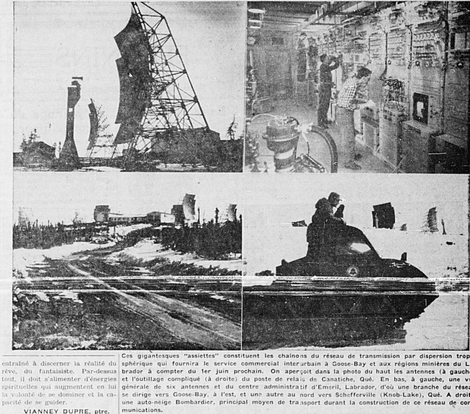
Ces gigantesques "assiettes" constituent les chainons du réseau de transmission par dispersion troposphérique qui fournira le service commercial interurbain à Goose-Bay et aux régions minières du Labrador à compter du 1er juin prochain. On aperçoit dans la photo du haut les antennes (à gauche) et l'outillage compliqué (à droite) du poste de relais de Canatiche, Qué. En bas, à gauche, une vue générale de six antennes et du centre administratif d'Emersil, Labrador, d'où une branche du réseau se dirige vers Goose-Bay, à l'est, et une autre au nord vers Schefferville (Knob-Lake), Qué. A droite une auto-neige Bombardier, principal moyen de transport durant la construction de ce réseau de communications.
