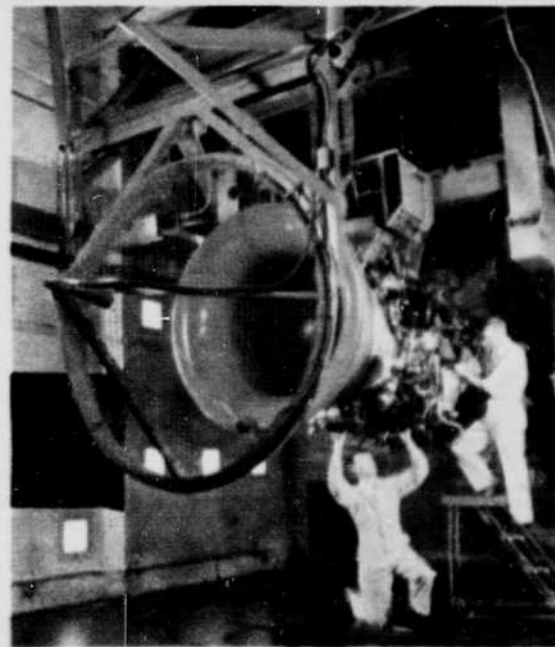
Dans l'une des deux sections du bâtiment, on vérifie le fonctionnement des puissants moteurs à réaction; des silencieux en atténuent le bruit. ✓
