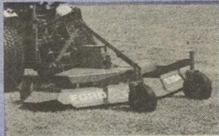
Tondeuses tractées, série 930A. Largeurs de coupe de 122, 150 et 183 cm. Hauteur de coupe réglable à 2,5 à 12,7 cm. Roues de calibrage. Tringlerie supérieure libre pour éviter de couper trop court.
