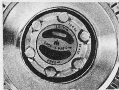
Moyeux bloquants automatiques. En 4 roues motrices, sans sortir du véhicule.
