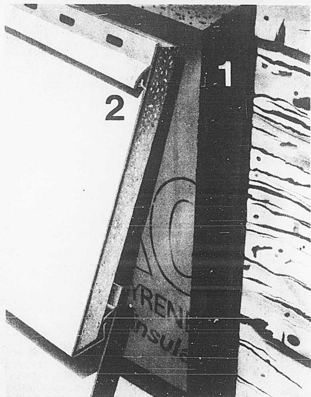
Les deux éléments constitutifs du duo Alcan: revêtement-super isolant, la feuille isolante de Styrofoam SM en bleu (1), puis, à l'extérieur, le revêtement d'aluminium renforcé Alcan (2).
