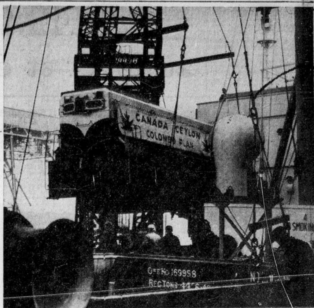
Pour le Ceylan — Cette immense grue mécanique transporte à bord du cargo "City of Leeds" une locomotive diesel de 71 tonnes, d'une valeur de $160.000. La scène se passe dans le port de Montréal. La locomotive est pour le Ceylan. Elle fait partie de l'aide de $2.000.000 en marchandises que le Canada a promis au plan Colombo. (Photo "PC")
