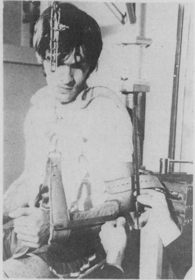
Assis à la chaise de contrôle Hettinger, un athlète subit un test ayant pour but de mesurer la force musculaire statique.
