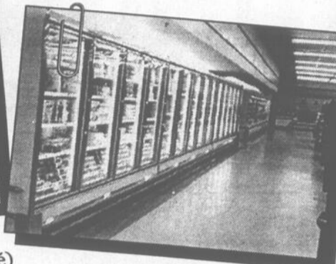
Congélateurs fermés pour crème glacée et desserts (espace doublé/14 portes)
