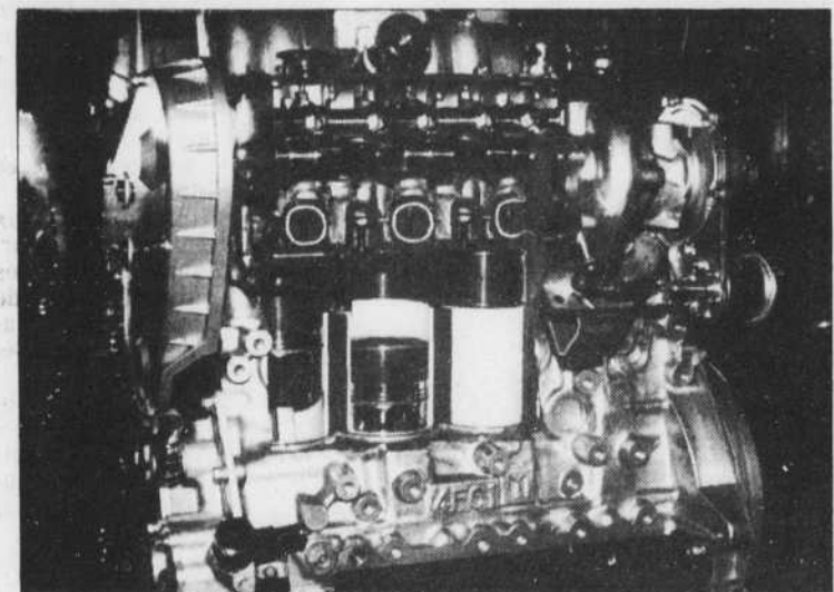
Dans le turbo-diesel de Isuzu, toutes les pièces exposées aux fortes températures sont recouvertes de céramique.
