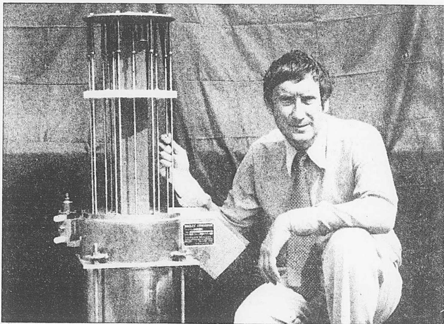
Richard Mozley, avec son équipement d'hydrocyclone. Il peut fonctionner avec une chaîne de traitement continu du minerai sans risque d'obstruction qui provoquerait un arrêt coûteux de toute la chaîne.
