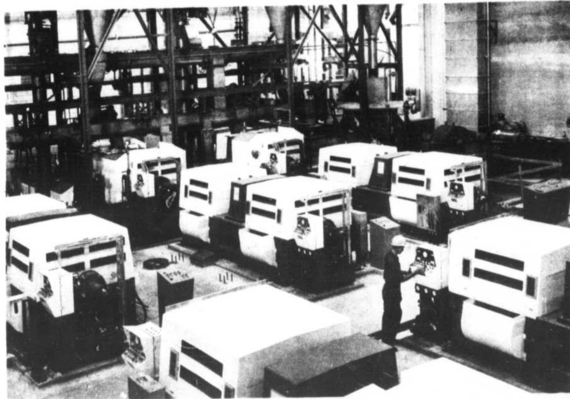
Les raffineuses à disques qui produisent la nouvelle pâte
