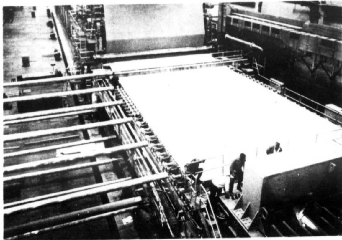
La section Fourdrinier de la machine, à son bout 'humide'
