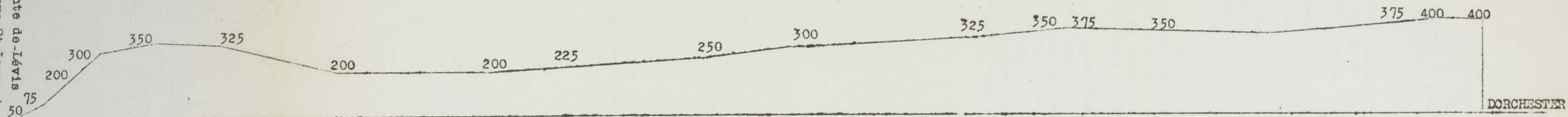
PROFIL TOPOGRAPHIQUE TRAVERSANT LE COMTE DE LEVIS DU NORD AU SUD EN SUIVANT LE 71° 10' de longitude
