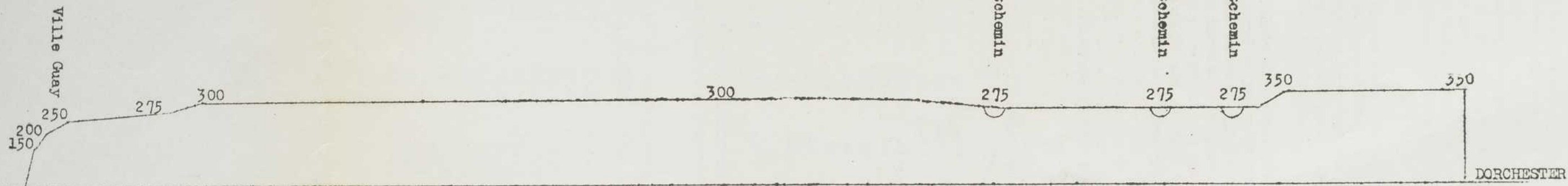
PROFIL TOPOGRAPHIQUE TRAVERSANT LE COMTE DE LEVIS DU NORD AU SUD EN SUIVANT LE 71° 5' DE LONGITUDE
