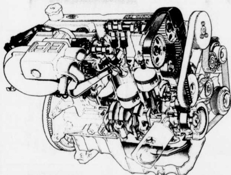
Le nouveau quatre cylindres Zeta disponible en Europe délivre 130 chevaux dans sa version de 1,8 litre. Des versions de ce moteur devraient équiper la prochaine génération de la Tempo.
